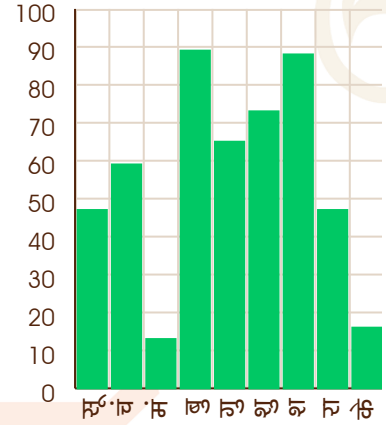
शनि - 27/11/2018
