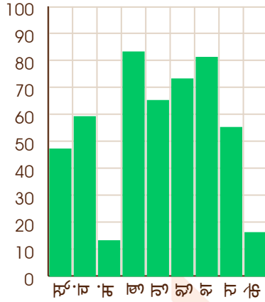
राहु - 27/11/1983
