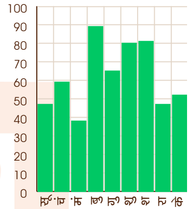
शुक्र - 27/11/2062
