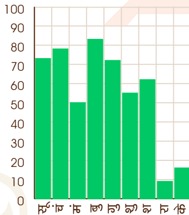
सूर्य - 27/11/2068
