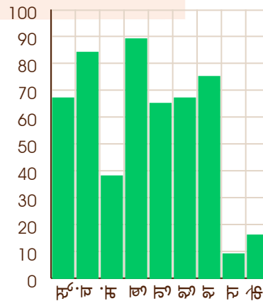
चन्द्र - 27/11/2078
