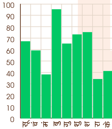
बुध - 27/11/2035
