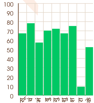
मंगल - 27/11/2085
