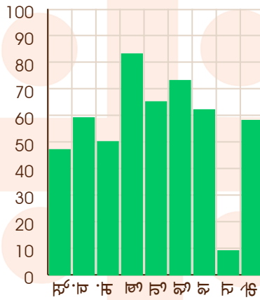
केतु - 27/11/2042
