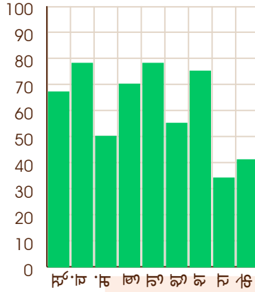
गुरु - 27/11/1999
