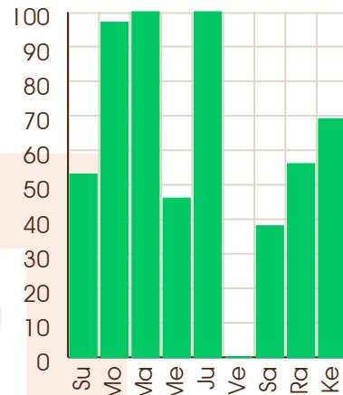
Mars - 05/08/2027
