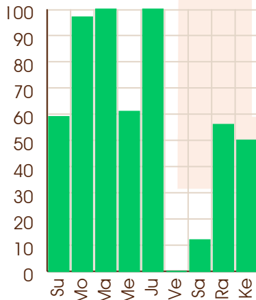
Sun - 05/08/2010
