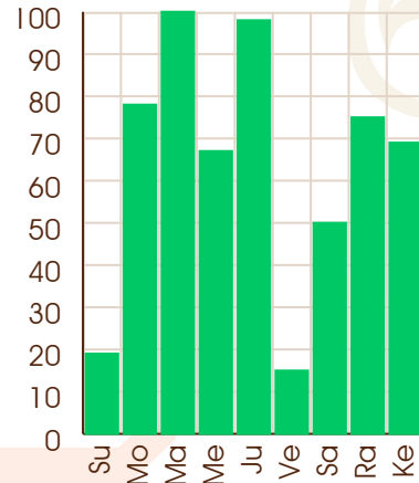
Venus - 05/08/2004
