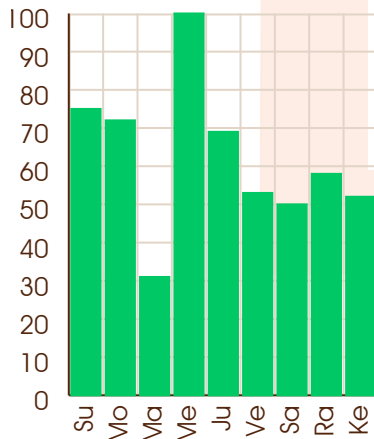
Sun - 08/07/2029
