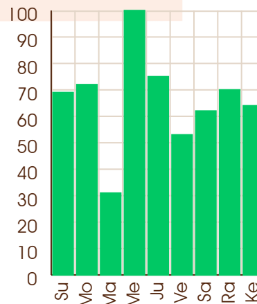
Jupiter - 08/07/2080
