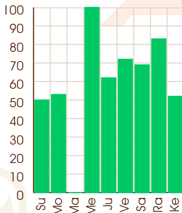
Rahu - 08/07/2064
