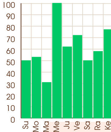
Ketu - 09/07/2003
