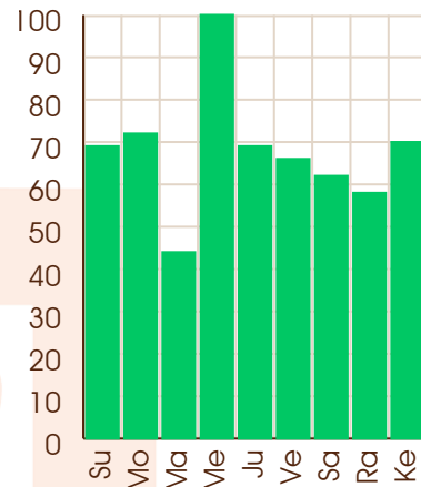
Mars - 09/07/2046
