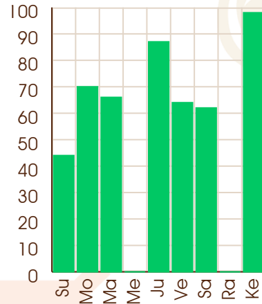
Ketu - 27/07/2055
