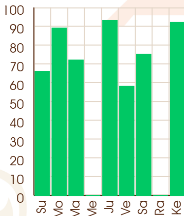
Mars - 27/07/2098
