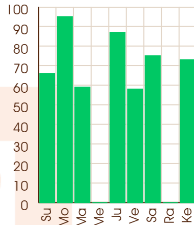
Moon - 27/07/2091
