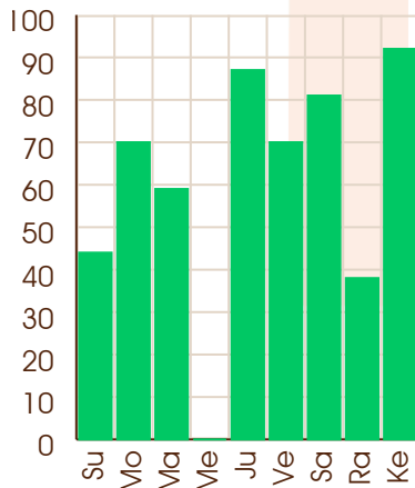
Venus - 27/07/2075
