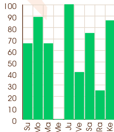
Jupiter - 27/07/2132
