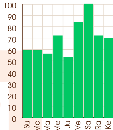
Mars - 26/09/2048
