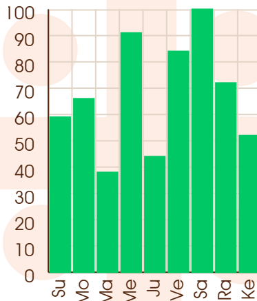
Moon - 27/09/2041
