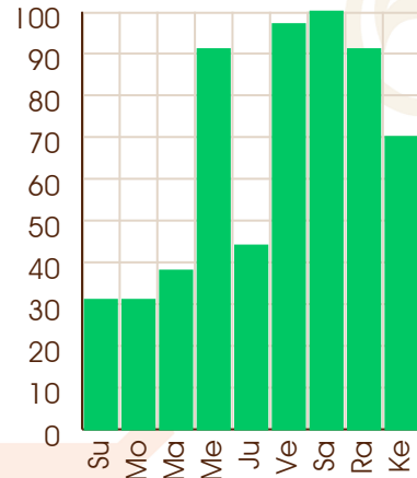
Venus - 27/09/2025
