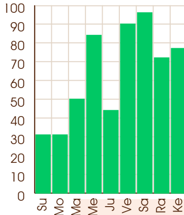
Ketu - 27/09/2005
