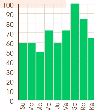
Jupiter - 27/09/2082
