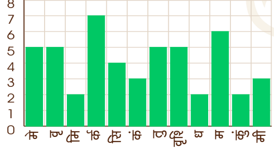
चन्द्र
