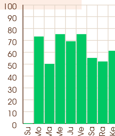
Mars - 18/02/2089
