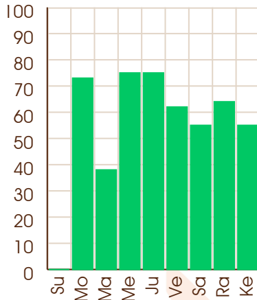
Jupiter - 19/02/2003
