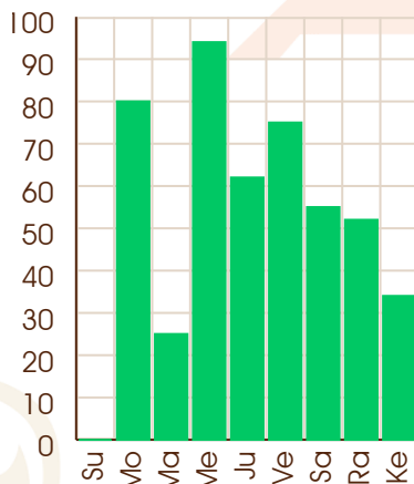
Moon - 19/02/2082
