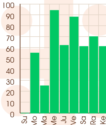
Venus - 19/02/2066
