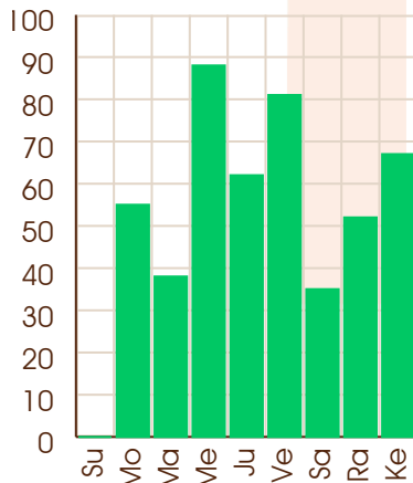
Ketu - 19/02/2046
