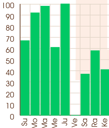
Sun - 03/04/2027
