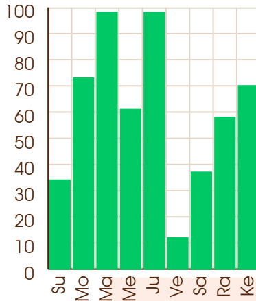
Ketu - 02/04/2001
