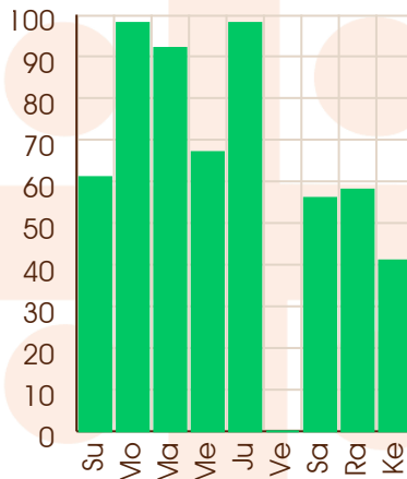
Moon - 02/04/2037
