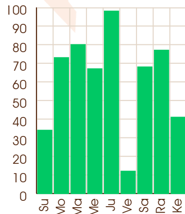
Saturn - 02/04/2097
