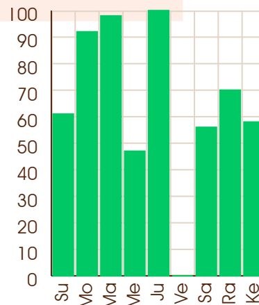
Jupiter - 02/04/2078
