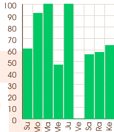
Mars - 02/04/2044
