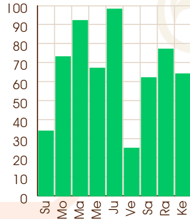
Venus - 02/04/2021
