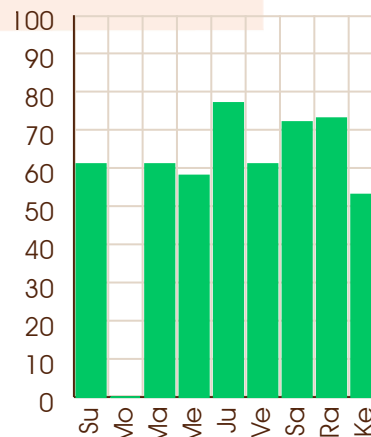
Mercury - 15/06/2093
