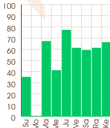
Ketu - 15/06/2100
