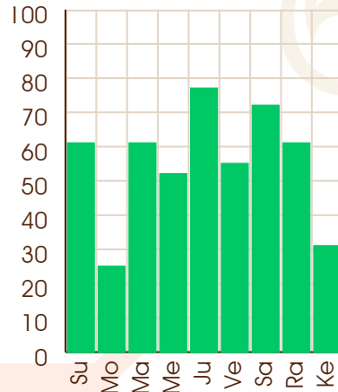
Moon - 14/06/2016
