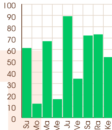
Jupiter - 15/06/2057
