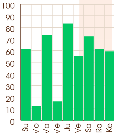
Mars - 15/06/2023
