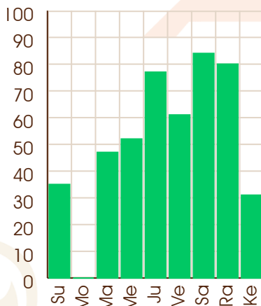
Saturn - 14/06/2076
