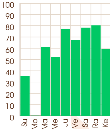
Venus - 14/06/2000
