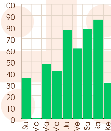
Rahu - 15/06/2041
