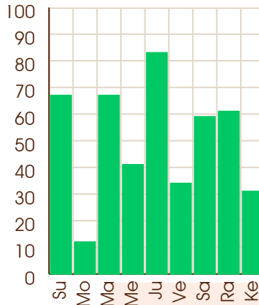
Sun - 15/06/2006
