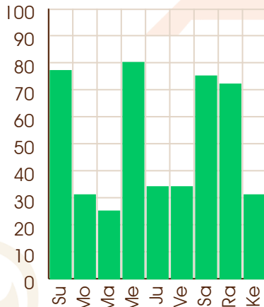
Jupiter - 01/02/2066
