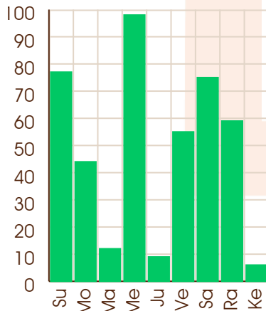
Moon - 01/02/2025
