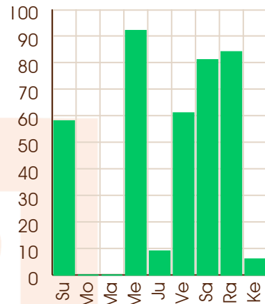
Rahu - 01/02/2050
