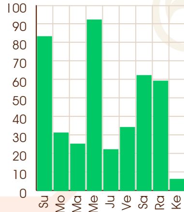
Sun - 01/02/2015
