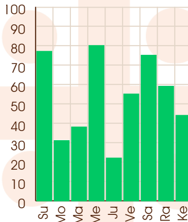
Mars - 01/02/2032
