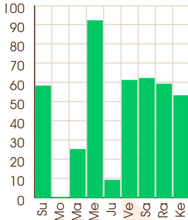
Ketu - 01/02/1989
