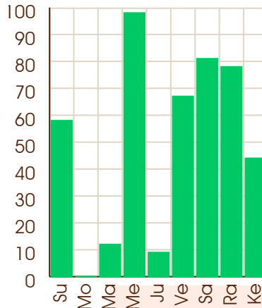
Venus - 01/02/2009
