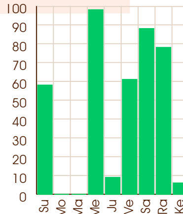
Saturn - 01/02/2085
