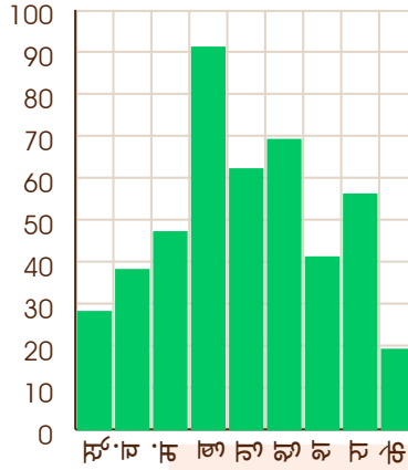
चन्द्र - 10/02/1999
