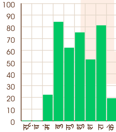
राहु - 10/02/2024
