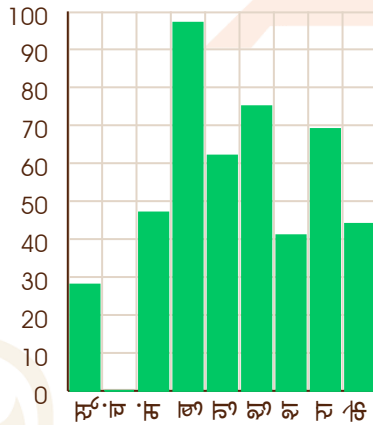
बुध - 10/02/2076
