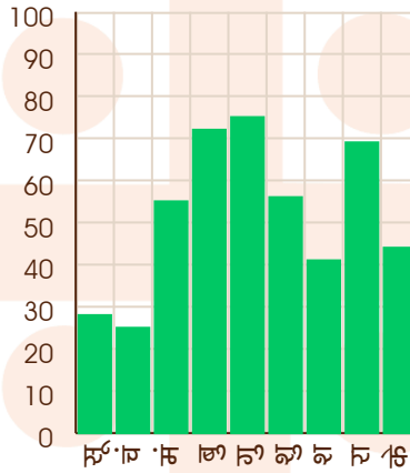
गुरु - 10/02/2040
