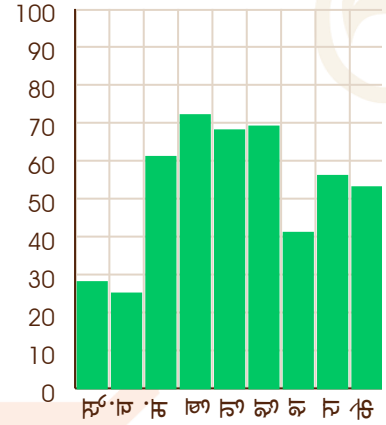
मंगल - 10/02/2006
