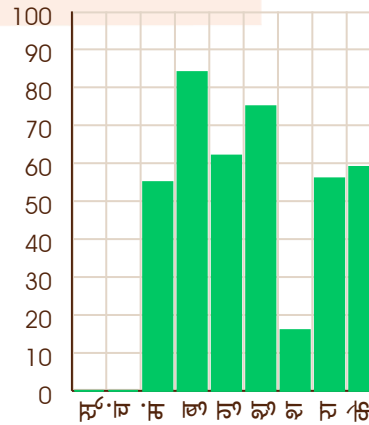
केतु - 10/02/2083
