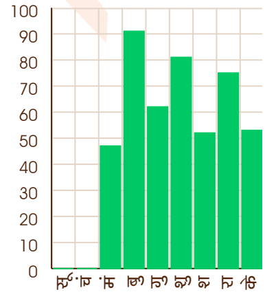
शुक्र - 11/02/2103
