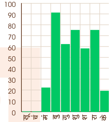
शनि - 10/02/2059
