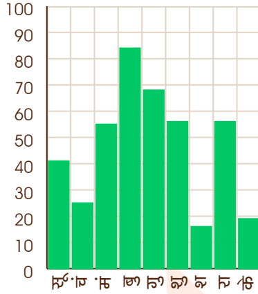
सूर्य - 09/02/1989
