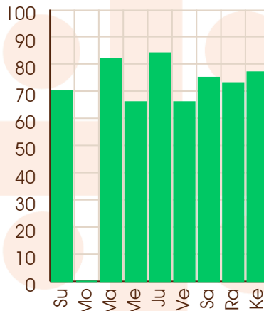
Venus - 07/07/2059
