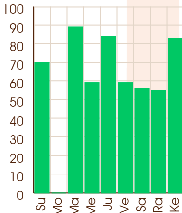
Ketu - 07/07/2039
