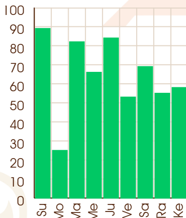
Moon - 07/07/2075
