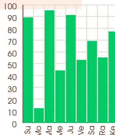
Mars - 06/07/2082
