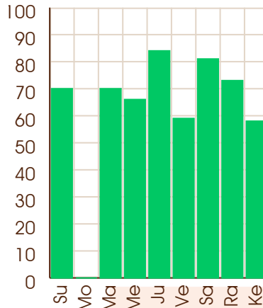
Saturn - 07/07/2015
