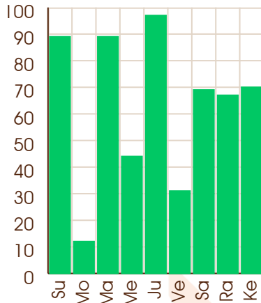
Jupiter - 06/07/1996
