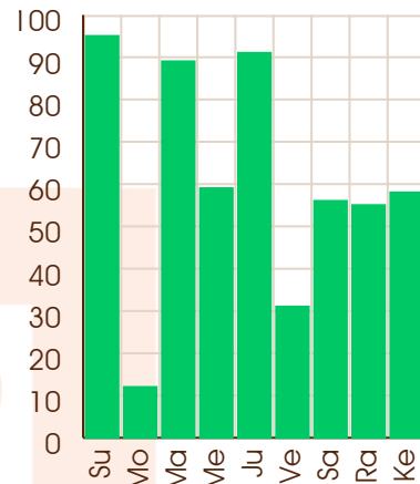
Sun - 06/07/2065
