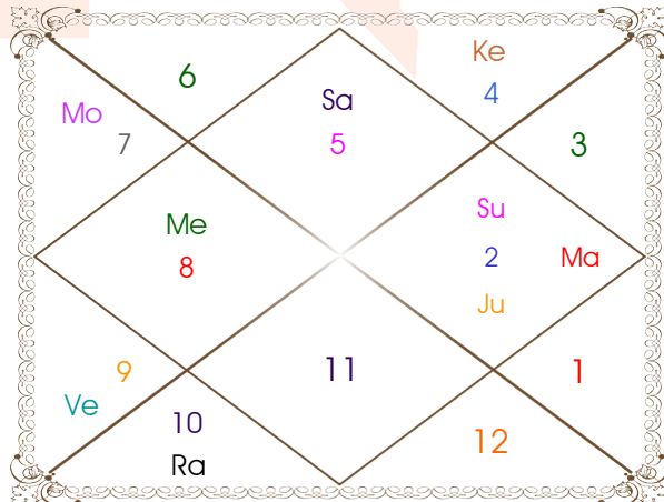
Shastiamsa Chart
