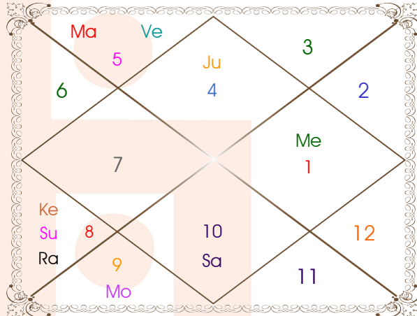
Khavedamsa Chart
