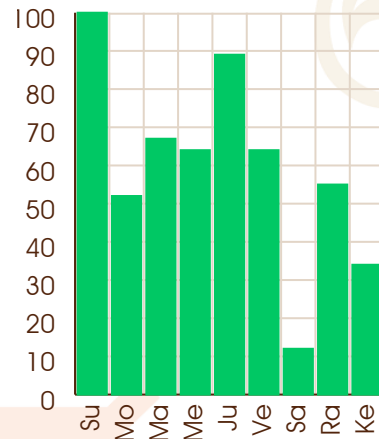
Jupiter - 30/11/2047
