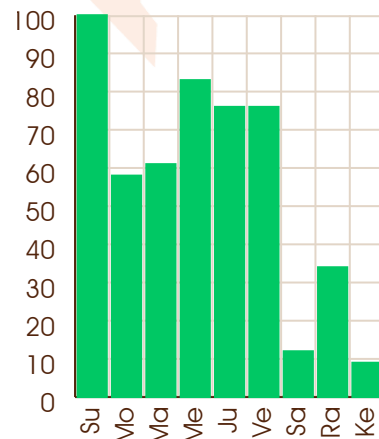
Moon - 01/12/2126
