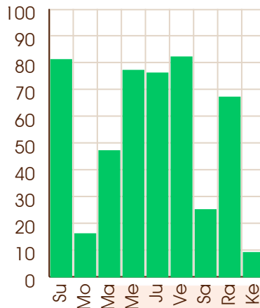
Rahu - 30/11/2031
