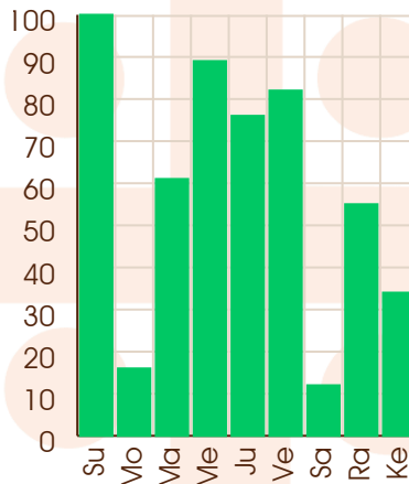
Mercury - 30/11/2083
