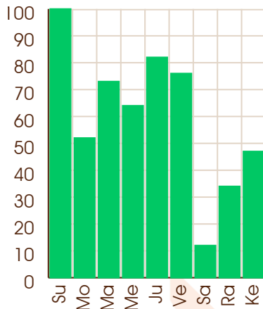
Mars - 30/11/2013
