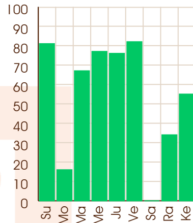
Ketu - 30/11/2090
