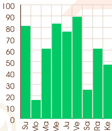
Venus - 01/12/2110
