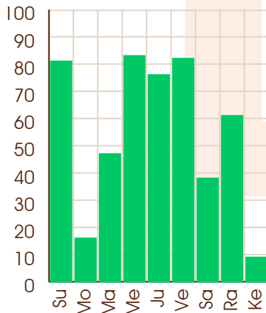
Saturn - 30/11/2066
