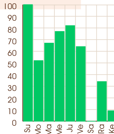
Sun - 01/12/2116
