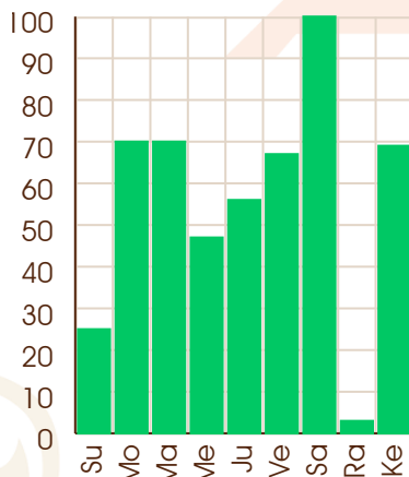
Mars - 21/02/2060
