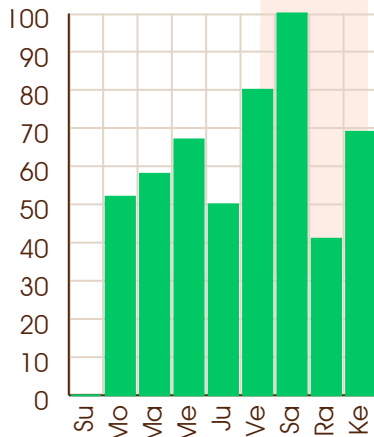
Venus - 20/02/2037
