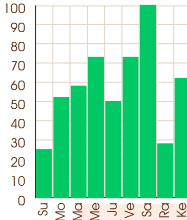
Mercury - 21/02/2010
