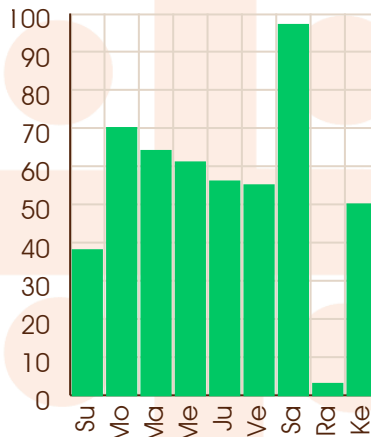
Sun - 21/02/2043
