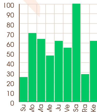
Jupiter - 21/02/2094
