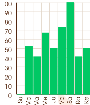
Saturn - 20/02/1993
