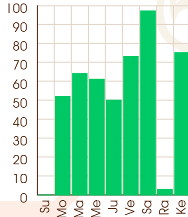
Ketu - 20/02/2017
