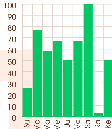
Moon - 20/02/2053
