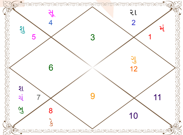
ષષ્ઠયંશ કુંડળી
