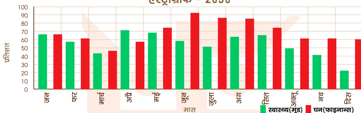
एस्ट्रोग्राफ - 2031
