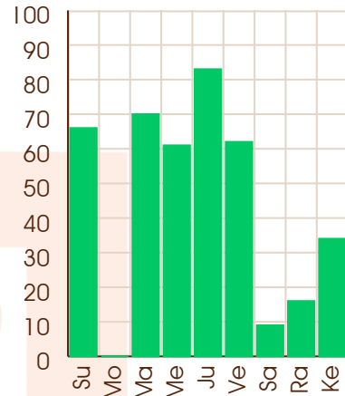
Ketu - 07/11/2048
