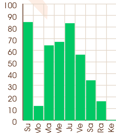
Moon - 07/11/2084
