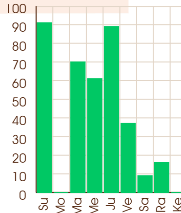
Sun - 07/11/2074
