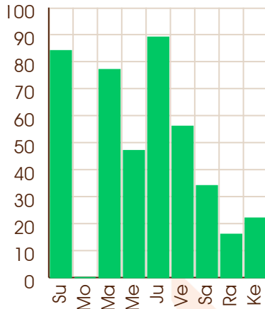
Mars - 08/11/1971
