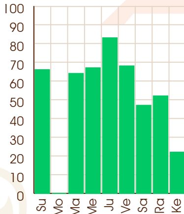
Venus - 07/11/2068
