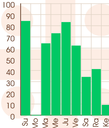
Mercury - 07/11/2041
