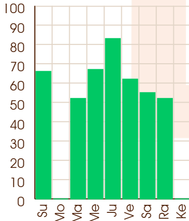
Saturn - 07/11/2024
