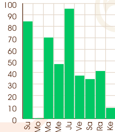
Jupiter - 07/11/2005
