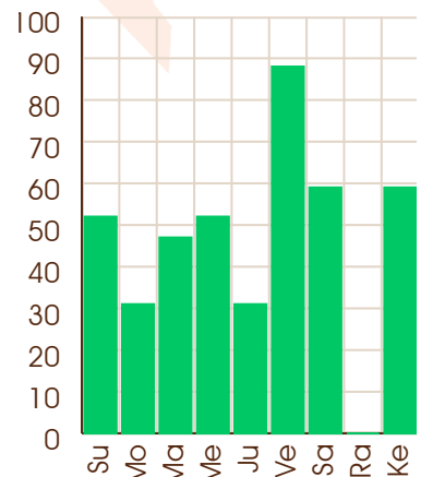
Mars - 31/01/2106
