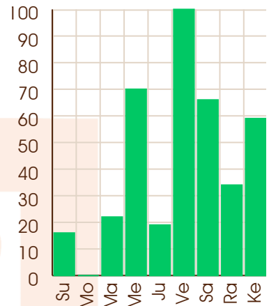
Venus - 31/01/2083
