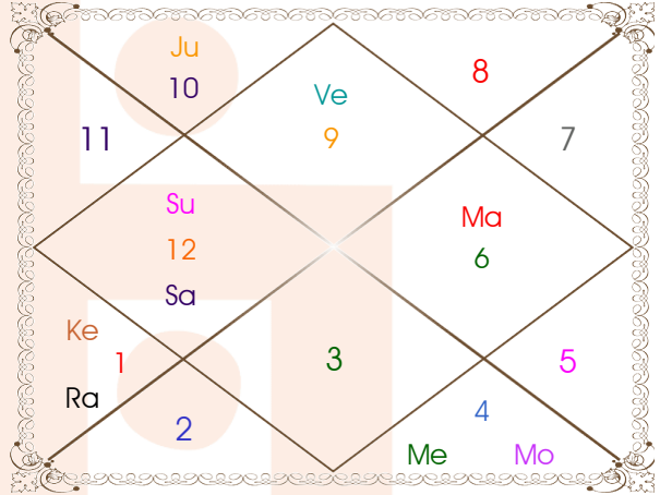
Khavedamsa Chart
