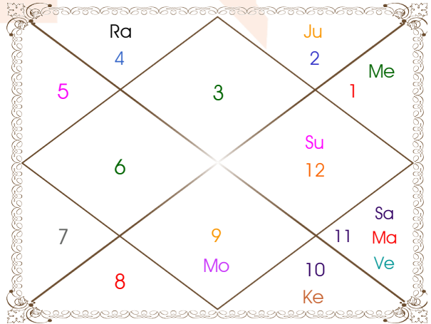
Shastiamsa Chart
