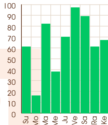
Mars - 25/07/2016
