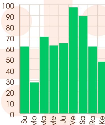
Moon - 26/07/2009
