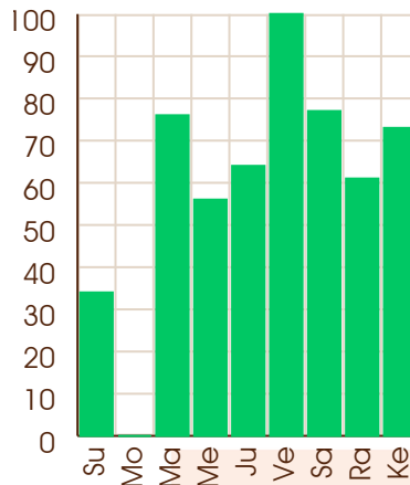
Ketu - 26/07/1973
